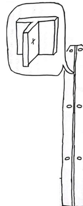
Poteau en fer en T section 35/40/5, 120 cm
