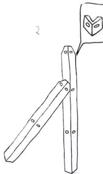
Poteau en fer en cornière avec jambe de force, section 35/20/35, 120 cm (X2)
